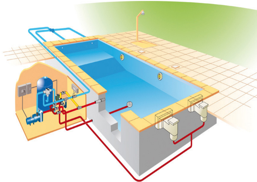
Schéma de principe d'une piscine traditionnelle avec projecteur. Automatisation : régulation pH, réchauffeur et surpresseur robot.
