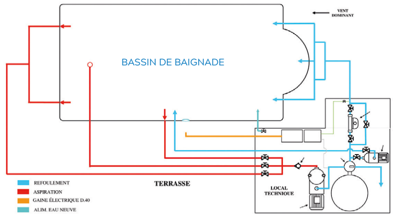
Schéma de principe d'une piscine traditionnelle avec projecteur. Automatisation : régulation pH, réchauffeur et surpresseur robot.
